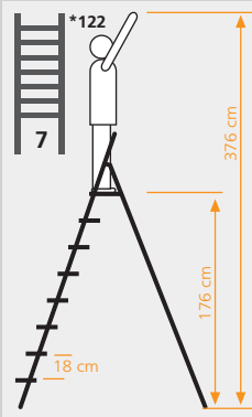
Yedi Basamaklı Merdiven Kullanım Boyutları
