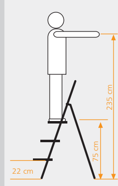
Üç Basamaklı Merdiven Kullanım Boyutları
