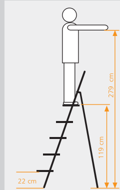
Beş Basamaklı Merdiven Kullanım Boyutları
