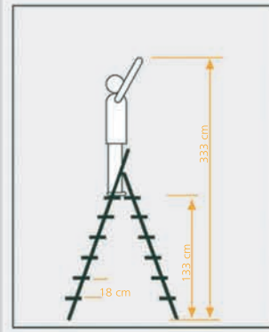
New Ağrı Altı Basamaklı Merdiven Kullanım Boyutları
