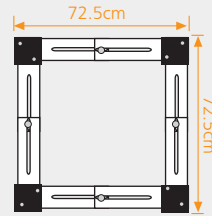
En Büyük Kare Ölçü
