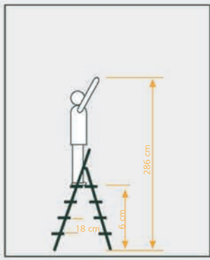
New Ağrı Dört Basamaklı Merdiven Kullanım Boyutları
