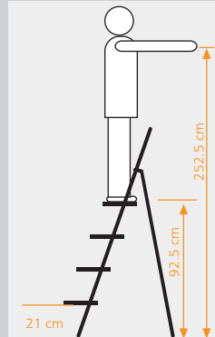
Dört Basamaklı Merdiven Kullanım Boyutları
