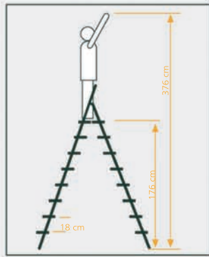
New Ağrı Sekiz Basamaklı Merdiven Kullanım Boyutları
