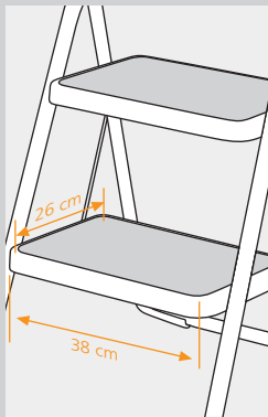
İki ve Üç Basamaklı Merdiven Ölçüleri
