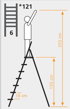
Altı Basamaklı Merdiven Kullanım Boyutları
