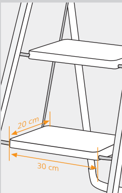
İkili, Üçlü, Dörtlü Merdiven Basamakları Ölçüleri
