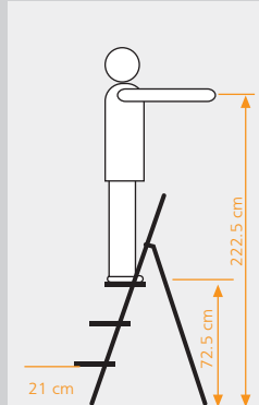
Üçlü Basamaklı Merdiven Kullanım Boyutları
